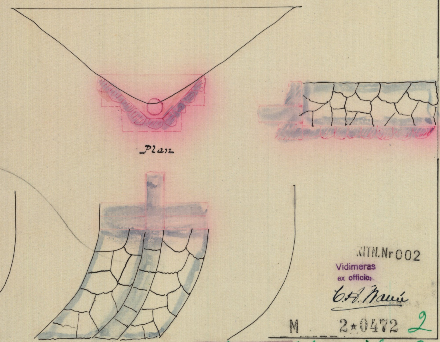
Förslag till ammurering af rör. 1:50
