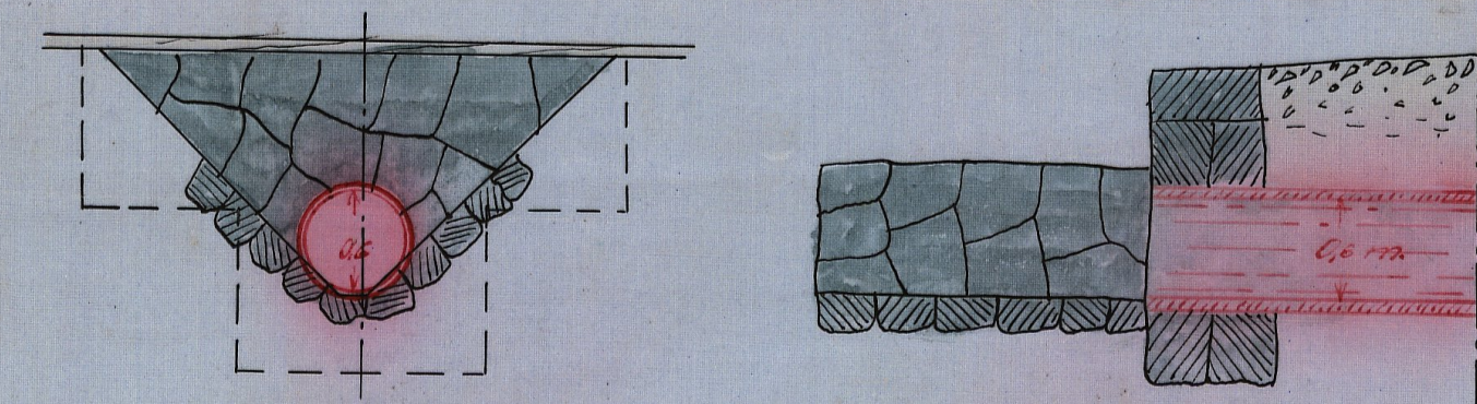
Förslag till ågavägsbro vid 16+2.
