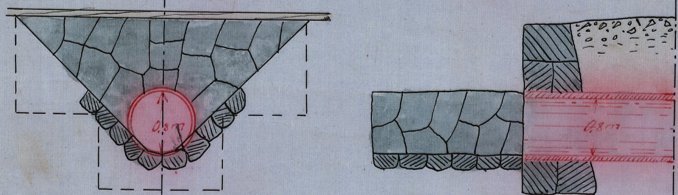
Förslag till bro för utfarsträgen vid 4+32.
