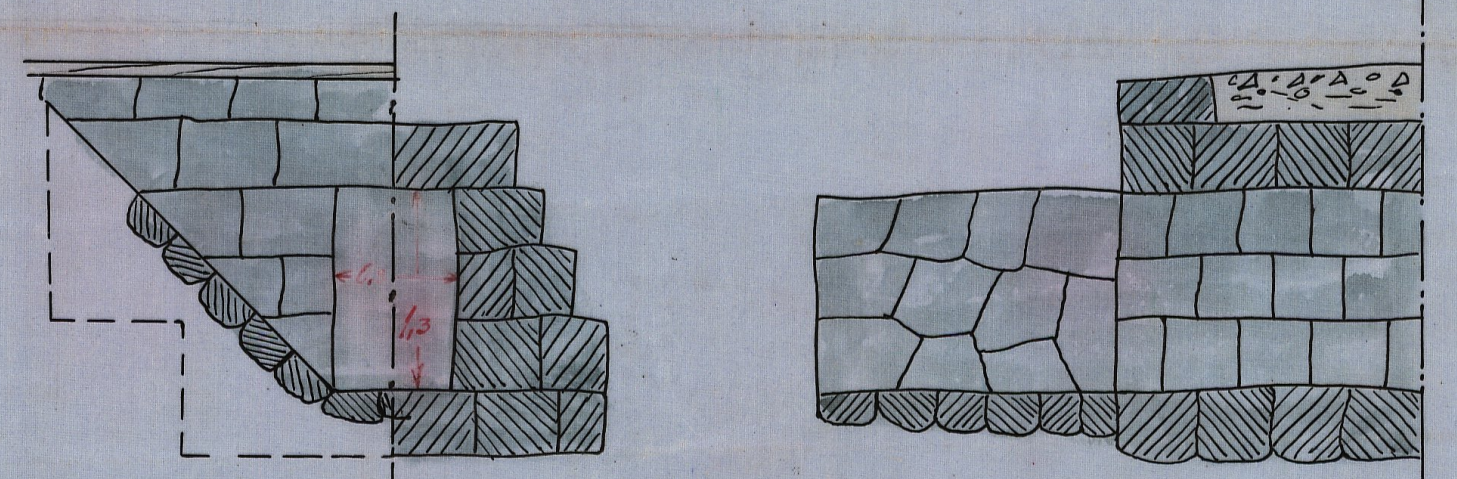
Förslag till ågavägsbro vid 4+32.
