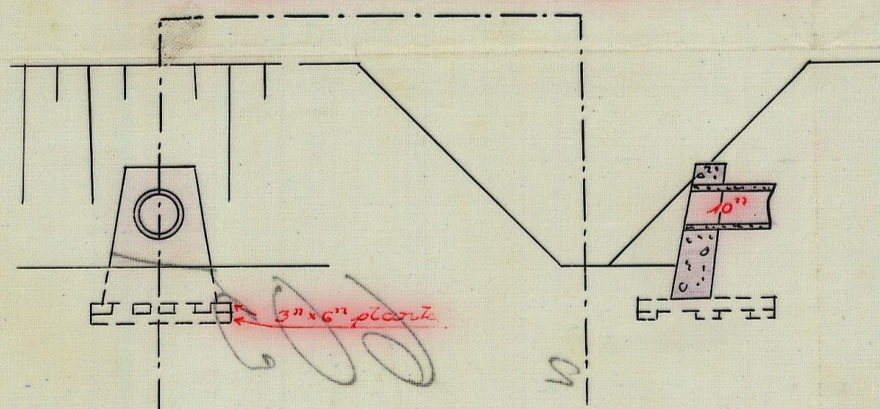
Förslag till rörutlapp vid A.
