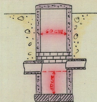
Typitning för brunnen:
