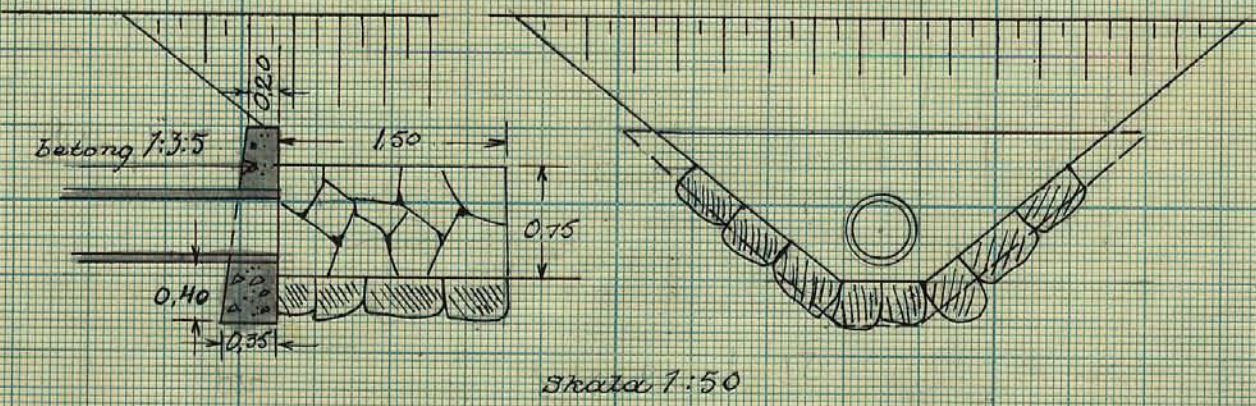
Rörutlopp vid sekt. 45+00
