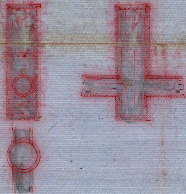
Förslag till brunn Skala 1:50
