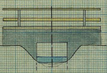
Trumma för allm. vägen Björka-Kropp's kyrka
