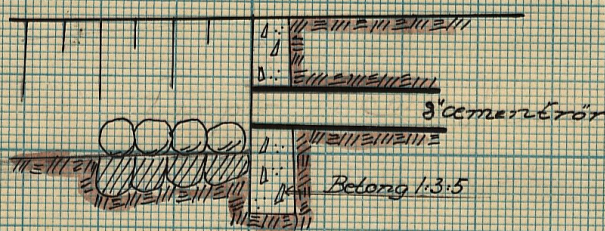
Rörutlopp vid sekt 0+00
