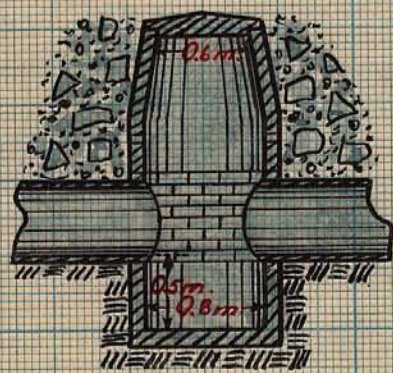
Typritning för brunn med 32" inre diameter.
