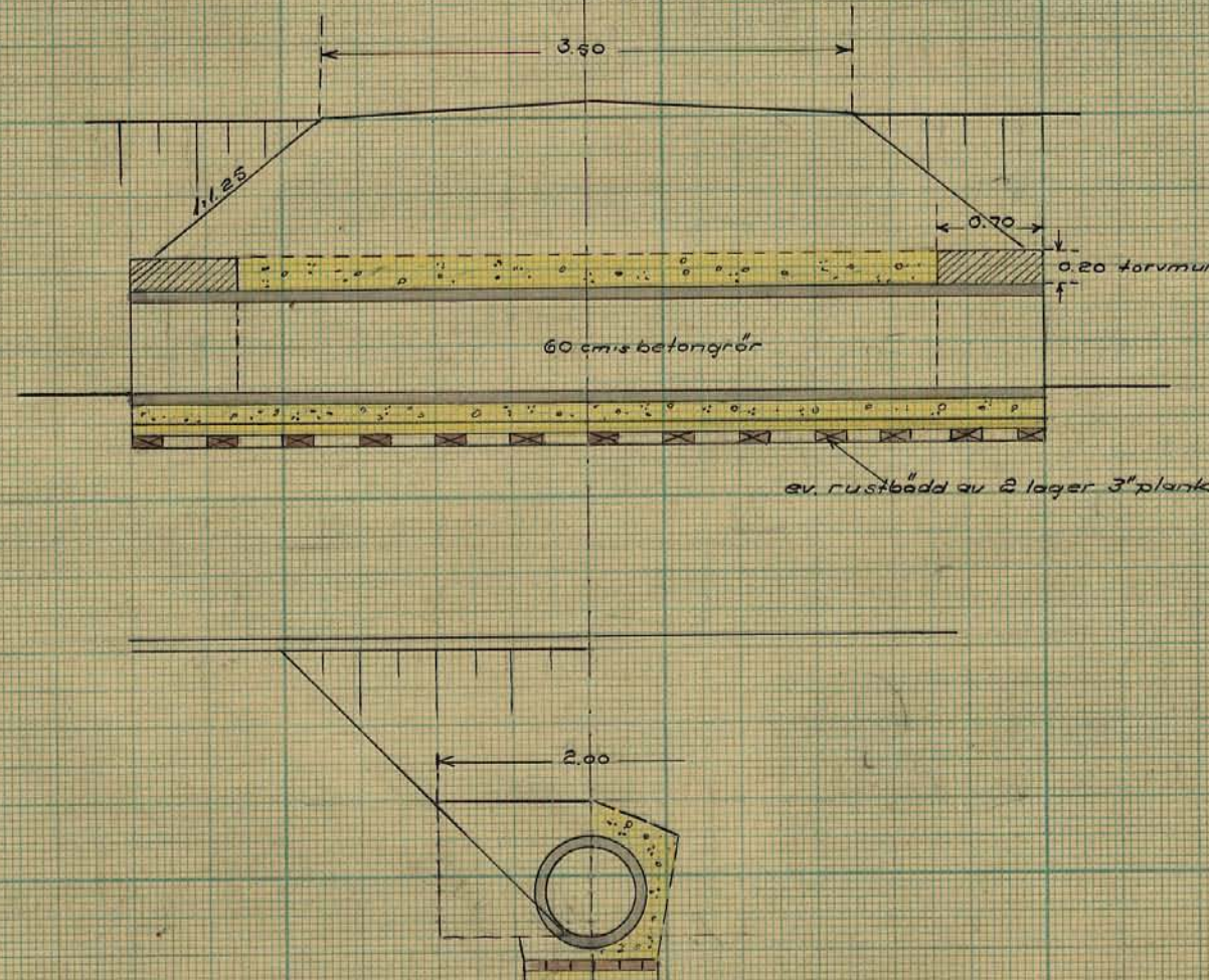
Ägövägsturmma vid sekt. 68+24. Skala 1:50.
