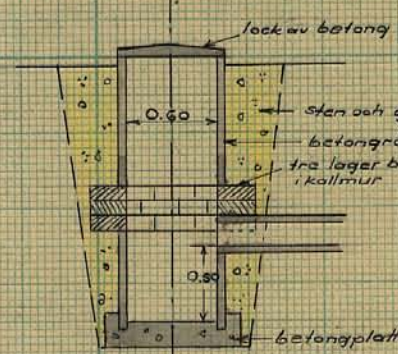
Brunn vid sekt. a Skala 1:50.
