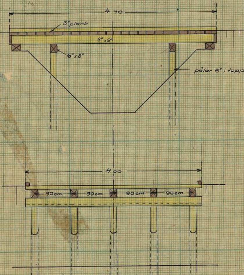
Typritning för broar av trä. Skala 1:50.
