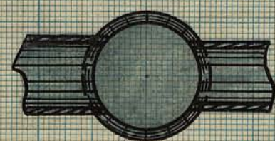
Typritning för brunn med 32" inre diameter. Skala 1:50.
