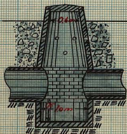
Typritning för brunn med 40" inre diameter. Skala 1:50.
