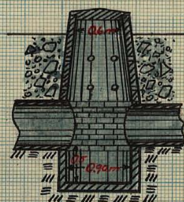
Typritning för brunn med 36" inre diameter. Skala 1:50.
