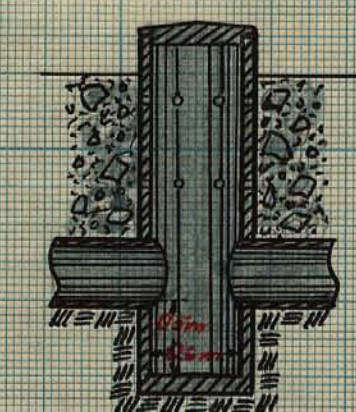
Typritning för brunn med 24" inre diameter. Skala 1:50.
