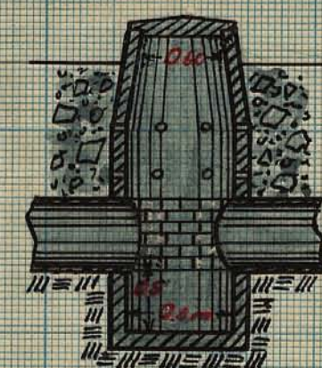
Typritning för brunn med 32" inre diameter. Skala 1:50.
