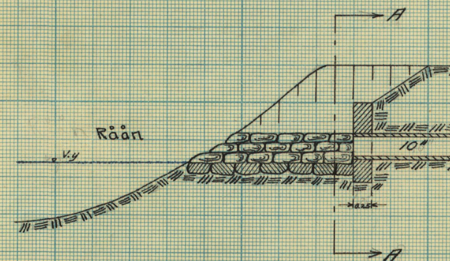
Längdsektion
