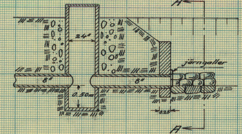
Skala 1:50 Längdsektion
