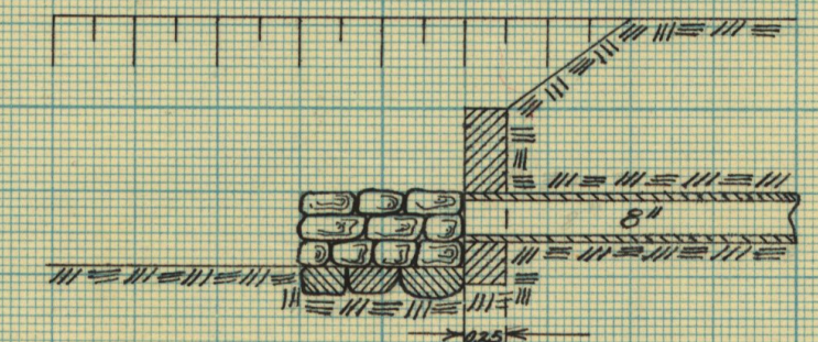
Frontvy
