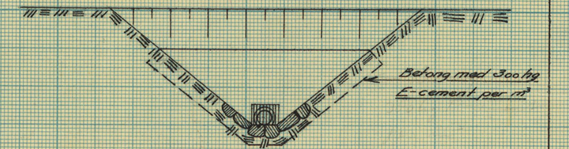
Sektion A-A
