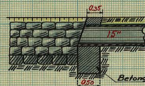
Typritning för ommurning vid 27+35
