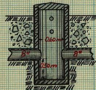
Typritning för brunn med 24" inre diameter. Skala 1:50.
