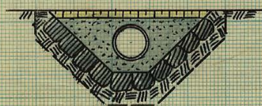
Typritning för ommurning vid 27+35
