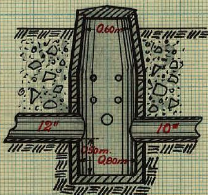
Typritning för brunn med 32" inre diameter. Skala 1:50.
