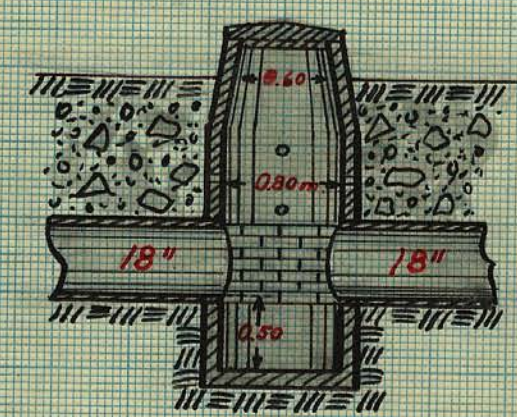
Typritning för brunn med 32" inre diameter. Skala 1:50
