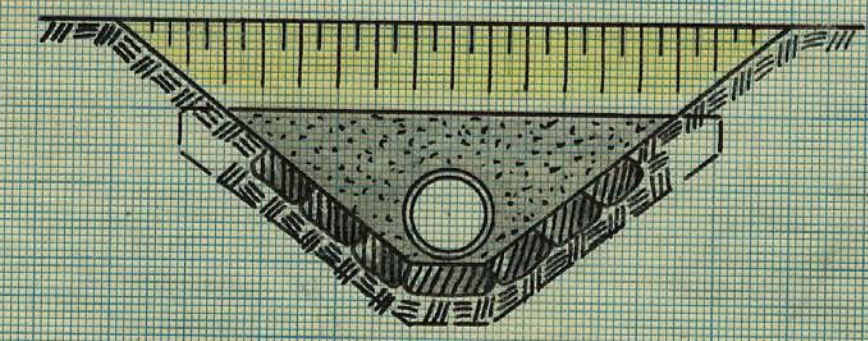
Typritning för ommurning av utloppet vid 5 Skala 1:50.
