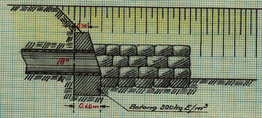
Typritning för ommurning av utloppet vid 5 Skala 1:50.
