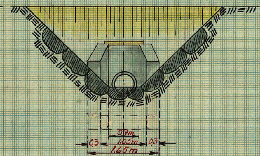
Typritning för intag vid 0
