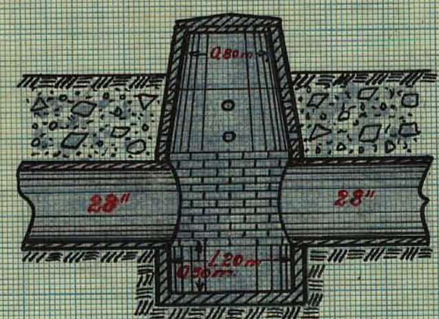
Typritning för brunn med 48" inre diameter.
