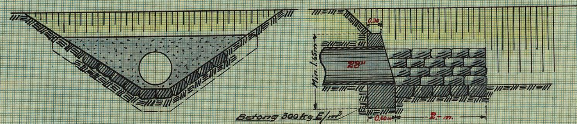
Typritning för ommurning vid 13+56
