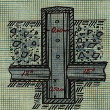
Typritningar för brunnar med 24" inre diameter.
