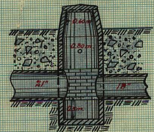
Typritningar för brunnar med 32" inre diameter.
