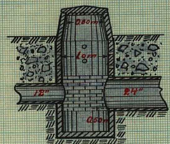
Typritning för brunn med 40" inre diameter.
