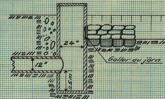
Förslag till brunn vid 4 Skala 1:50
