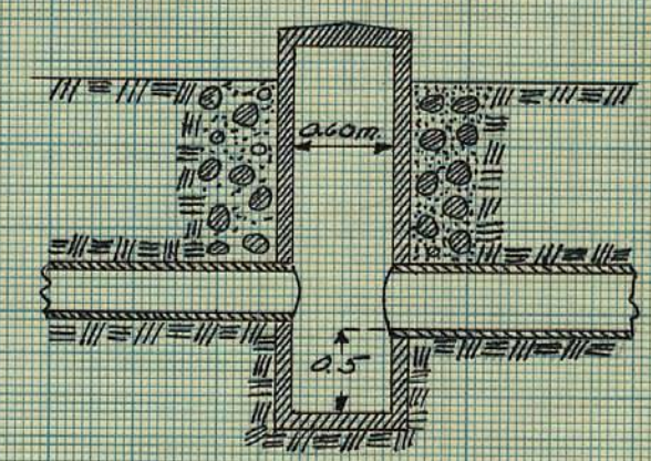
Typritning för brunnar Skala 1:50
