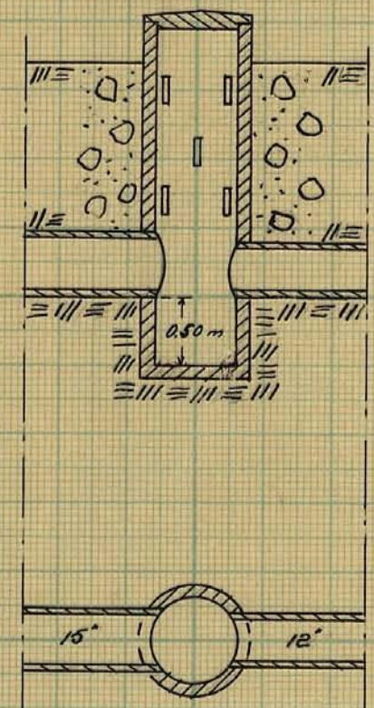
Förslag till 24" brunn Skala 1:50
