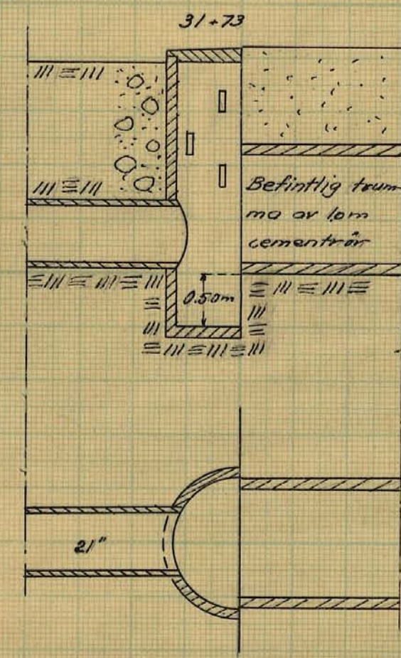
Förslag till 48" anslutningsbrunnar vid 31+48 och 31+73 Skala 1:50
