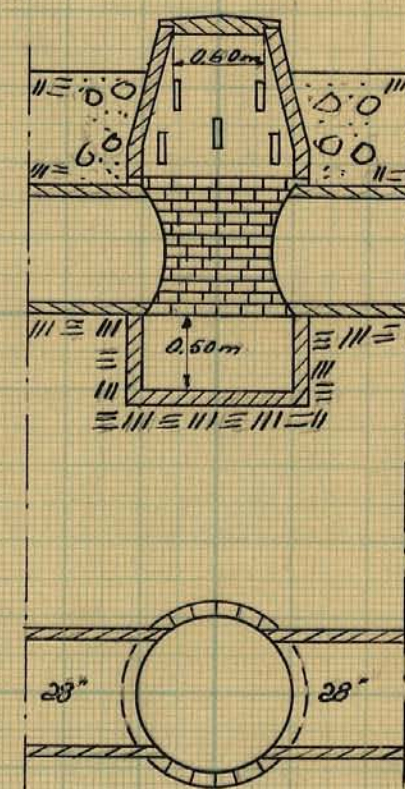
Förslag till 40" brunn Skala 1:50
