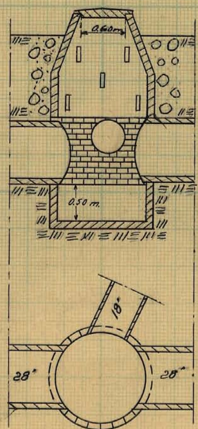
Förslag till 48" brunn vid 3+33 Skala 1:50
