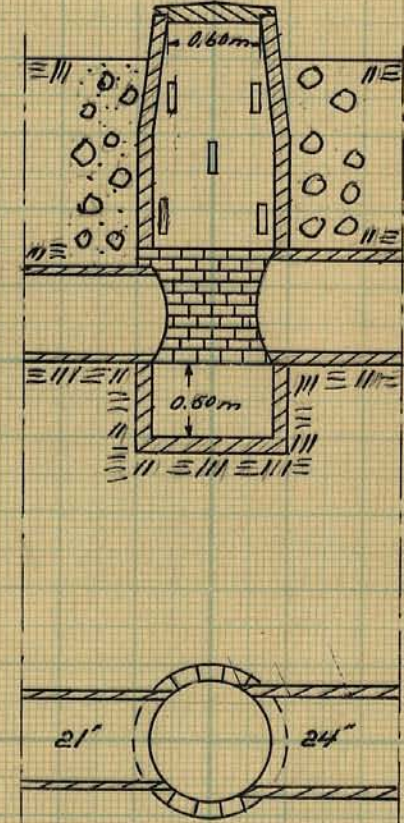
Förslag till 32" brunn Skala 1:50
