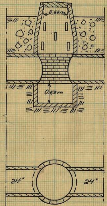
Förslag till 36" brunn Skala 1:50
