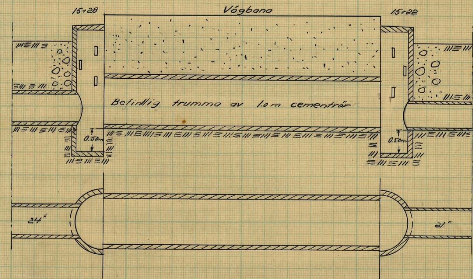
Förslag till 48" anslutningsbrunnar vid 15+22 och 15+28 Skala 1:50
