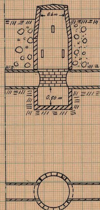
Förslag till 32" brunn
