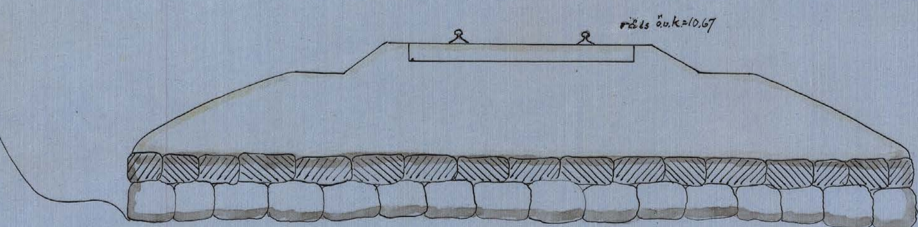
Järnvägstrumma under Håningsborg-Engelholms järnväg skala 1:50
