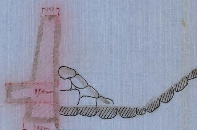
Förslag till kringmurning av utloppet vid E skala 1:50
