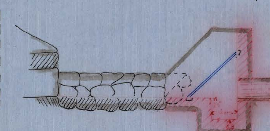
Förslag till Intag vid D skala 1:50
