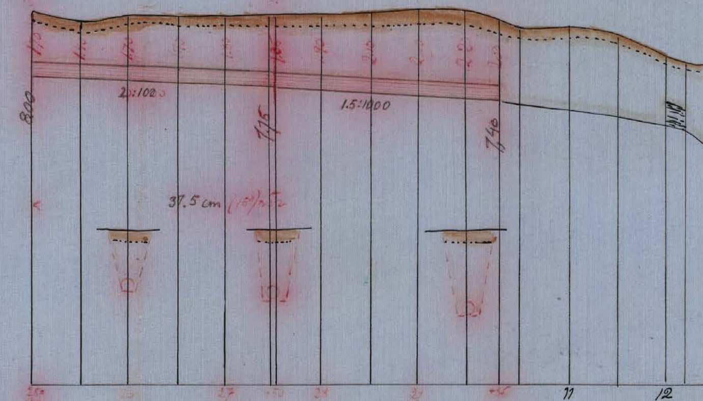
Kringmurning av utloppet vid E sektion vid A-A skala 1:50
