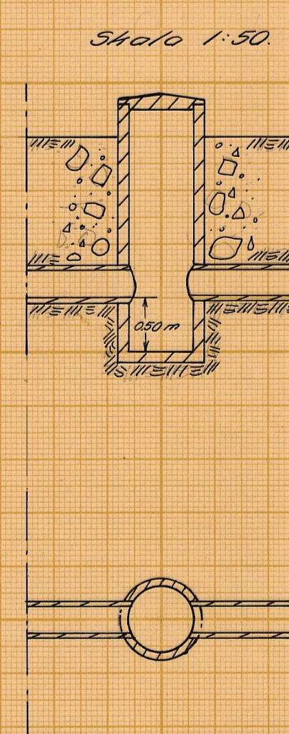
Förslag till 24" brunn.
