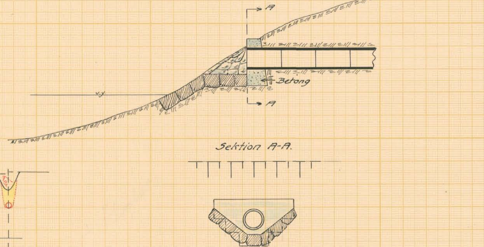
Typritning för rörutlopp Skala 1:50
